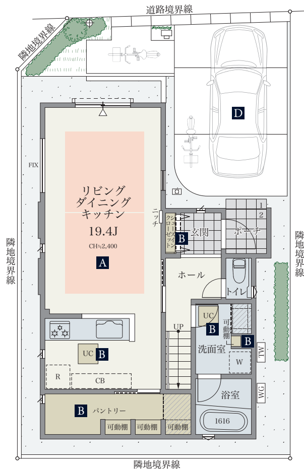
【1F】
